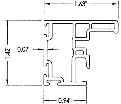
5 STILE
